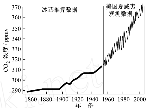
图5 150年来大气中CO 2 浓度变化 [3]
