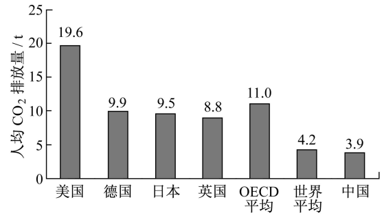
图 12 人均 CO_2 排放量国际比较 ⑮
