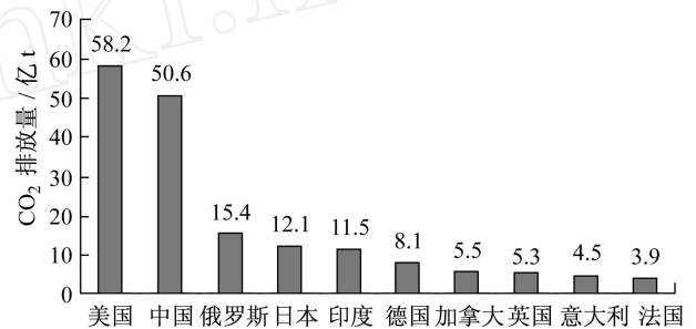
图 13 主要国家燃料燃烧 CO_2 排放情况 ⑯
