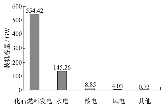
图18 2007年我国电力装机容量 ②
